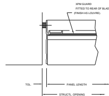
560. JAMB DETAIL
