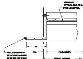
552. JAMB DETAIL
